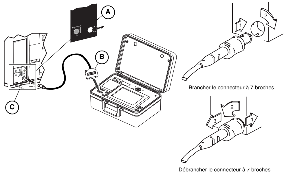
Figure 3 – Raccordement aux déclencheurs Micrologic et ET
