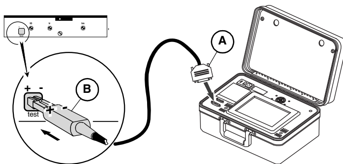
Figure 2 – Raccordement aux déclencheurs STR
